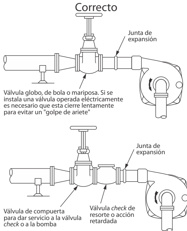
Figura 6 Tubería de descarga
